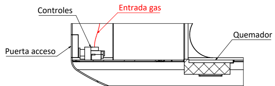
DETALLE B ESCALA 1 : 10
