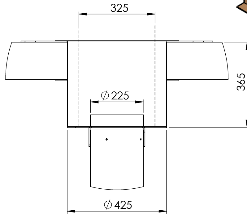
DETALE B SCALA 1 : 10
